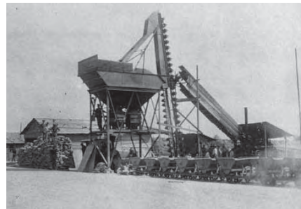
Nelle due foto, l'Autostrada MI-TO, costruzione casello Rho, 17 settembre 1932
