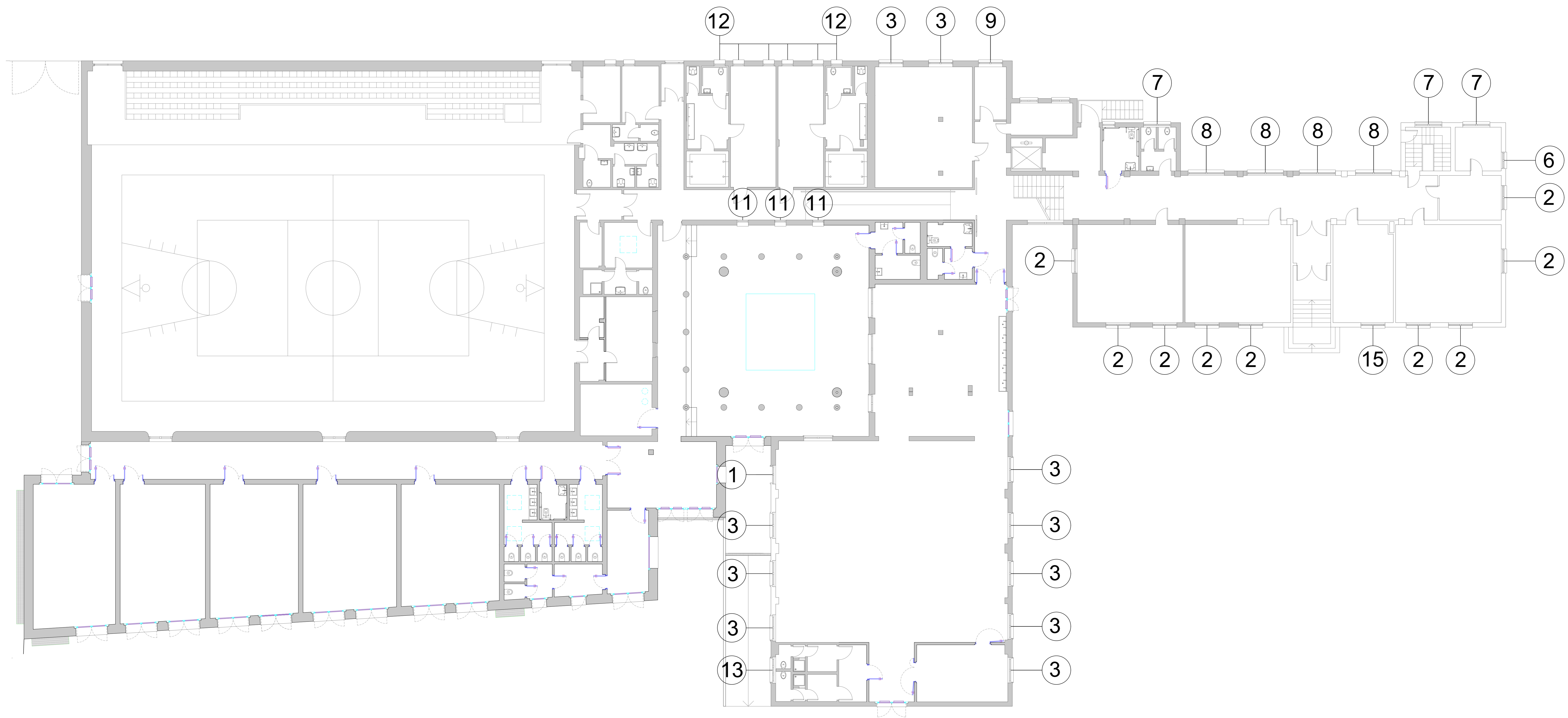
Pianta piano terra
