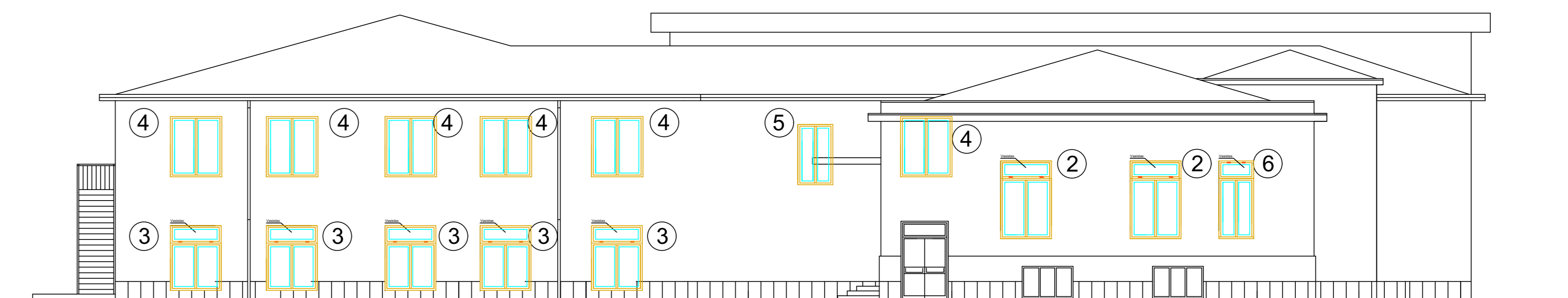
PROSPETTO D - D
