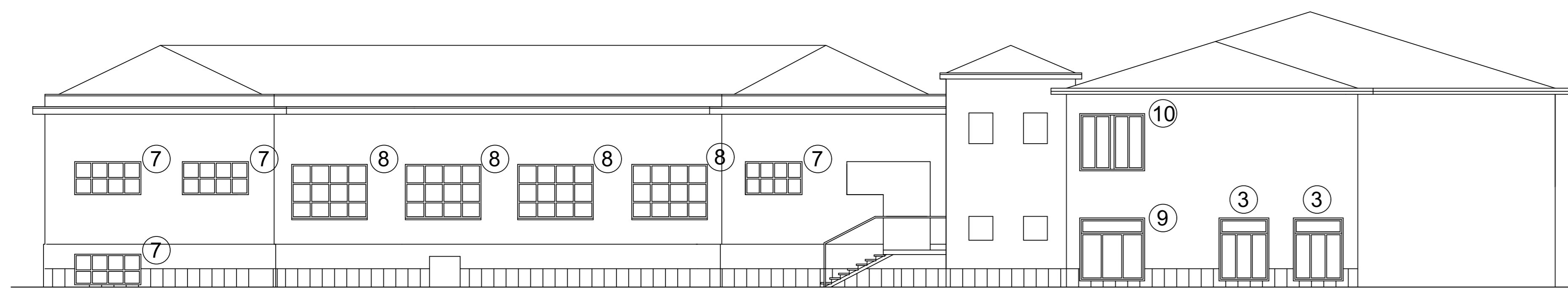
PROSPETTO C - C STATO DI FATTO
